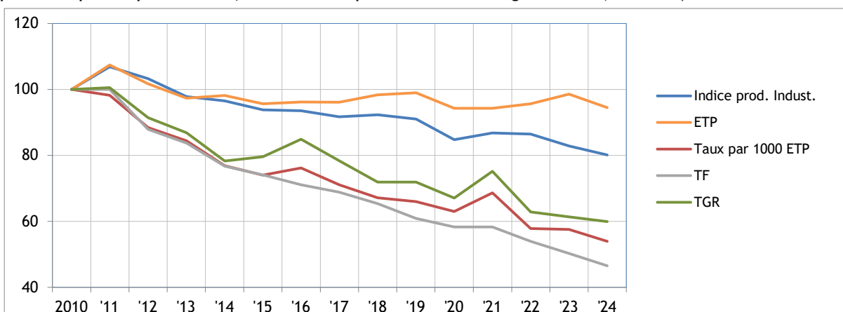
6. Evolution de 2010 à 2024 de l'indice de production industrielle, de l'emploi (ETP), du taux des accidents avec plus de 30 jours d'incapacité temporaire par 1000 ETP, du taux de fréquence et du taux de gravité réel (2010=100)
